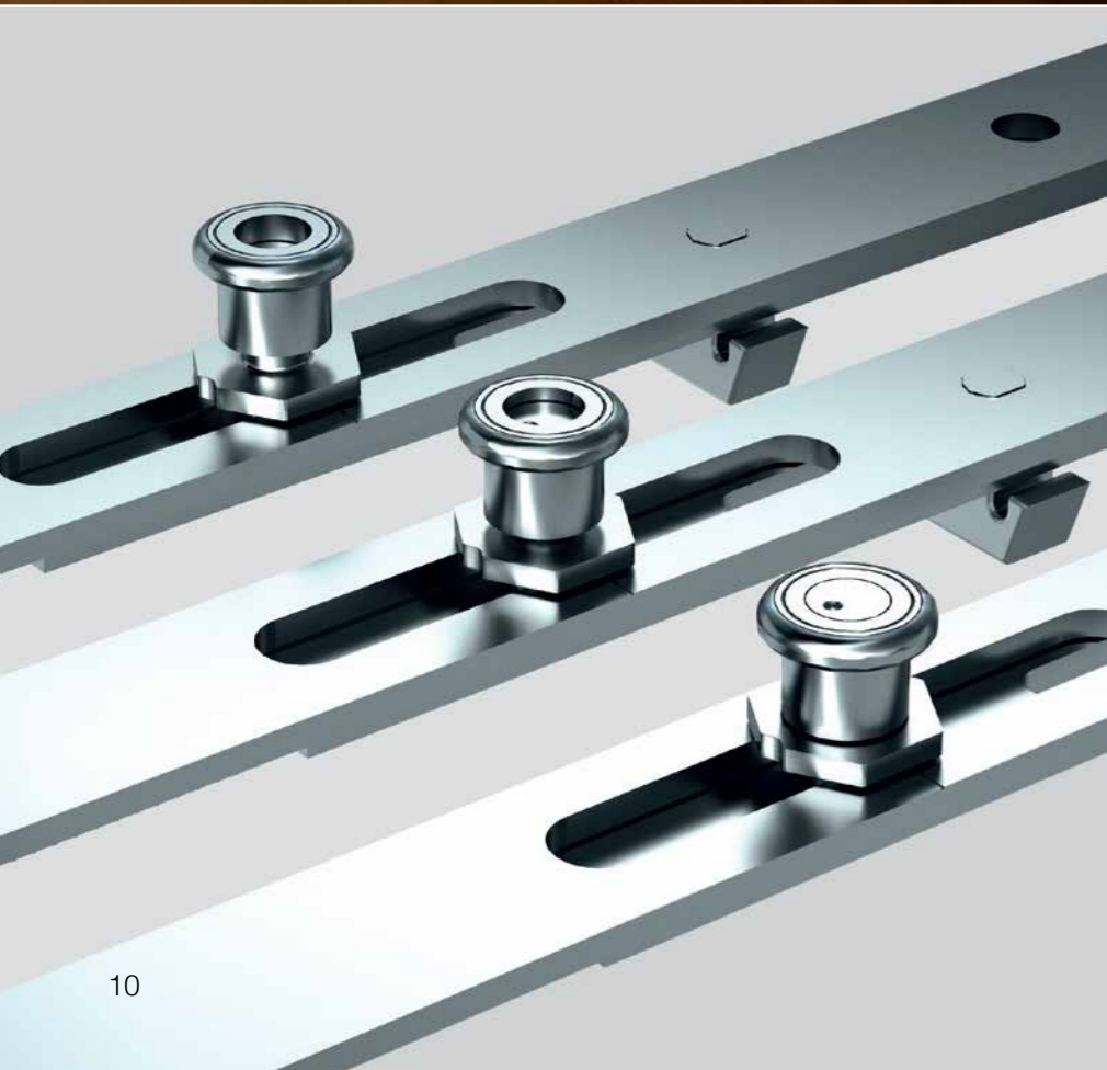
Particolare della ferramenta antieffrazione
