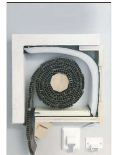
Art. 021 Campione del sistema Renova per la coibentazione del Cassonetto ISPEZIONE FRONTALE Prezzo unitario € 85
